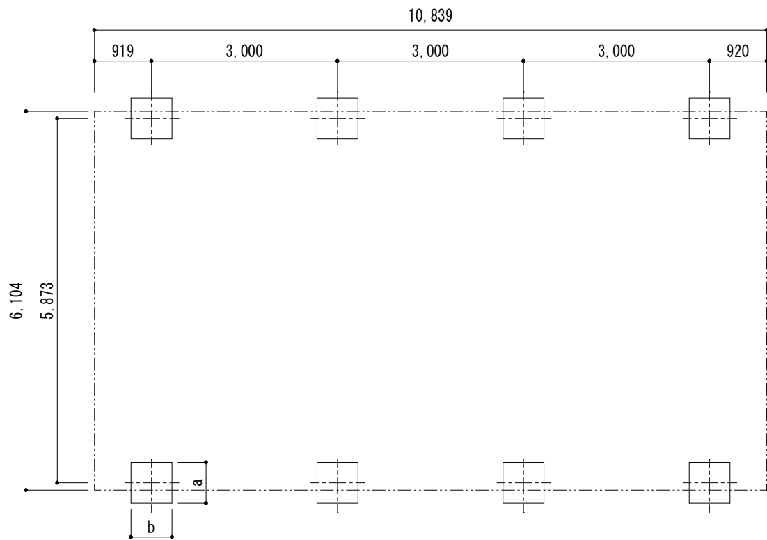
■基礎配置図
